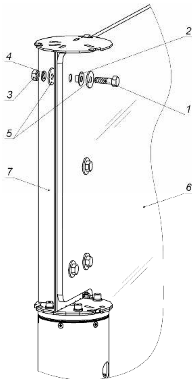
Рисунок 12. Установка створки
