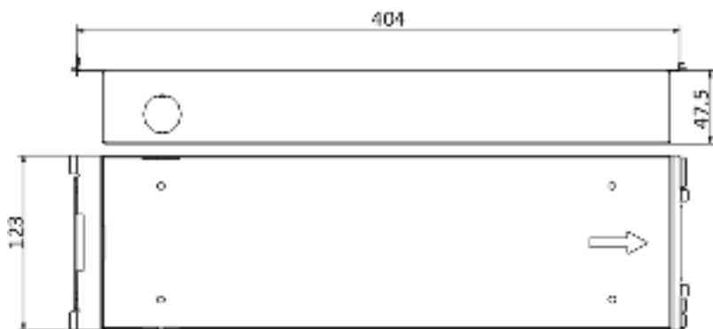
Рисунок 5-1 Вид спереди и сбоку
