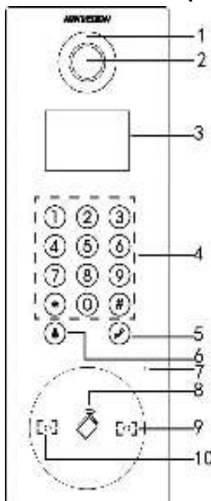
Рисунок 2-1 Передняя панель DS-KD8102-V
