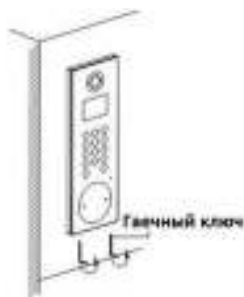
Рисунок 5-5 Затягивание винтов вызывной панели
