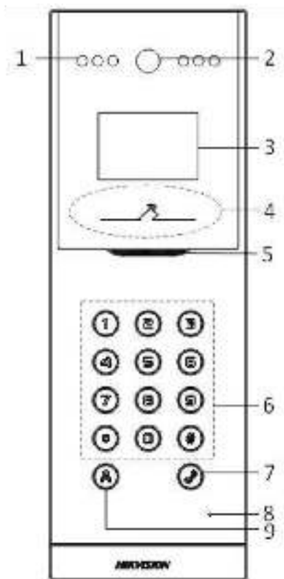
Рисунок 2-3 Передняя панель DS-KD8002-VM
