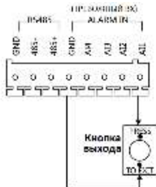
Рисунок 5-22 Подключение кнопки выхода для модели DS-KD6002-VM
