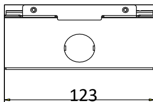
Рисунок 5-2 Вид сверху
