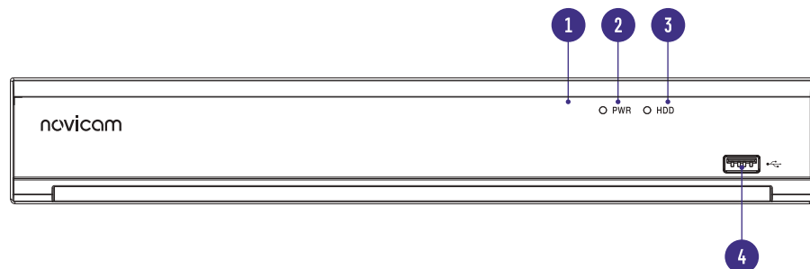
Рис. 3 Интерфейс передней панели SMART 1804 | SMART 1808 | SMART 1816
