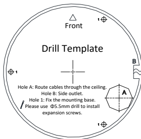
Рисунок 2-6 Шаблон крепления (камера II типа)
