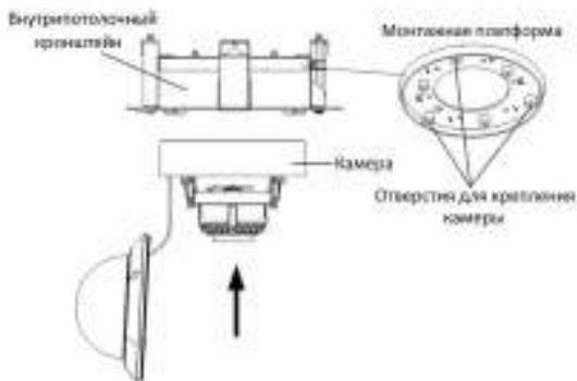
Рисунок 2-14 Установка камеры на монтажную платформу
