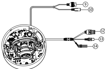
Рисунок 1-4 Кабель камеры I типа (2)
