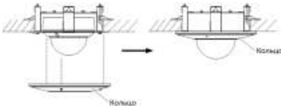
Рисунок 2-17 Установка кольца
