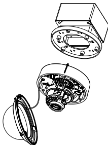
Рисунок 2-29 Установка камеры
