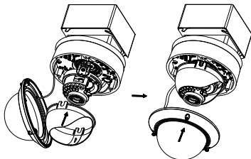
Рисунок 2-30 Установка защитного кожуха и купола
