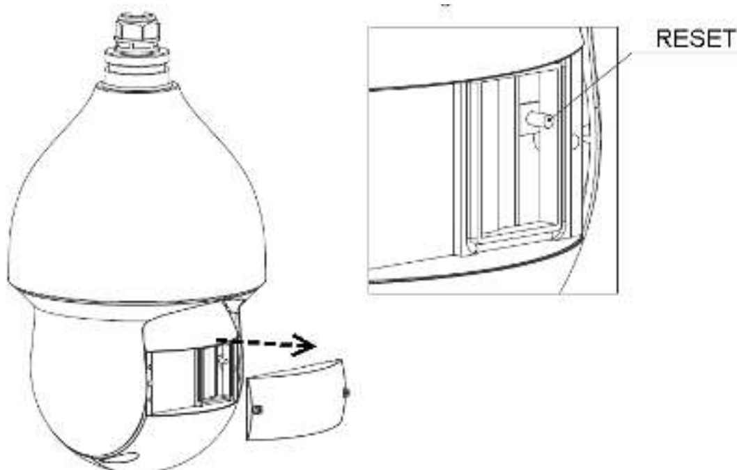
Рис. 9 Кнопка сброса на заводские параметры
