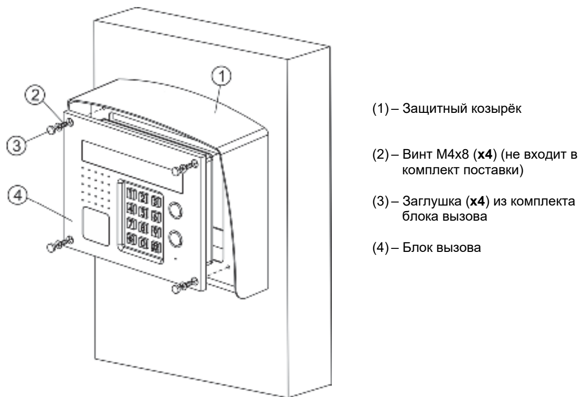
Рисунок 6.3 - Установка блока вызова на монтажный комплект МК-432
