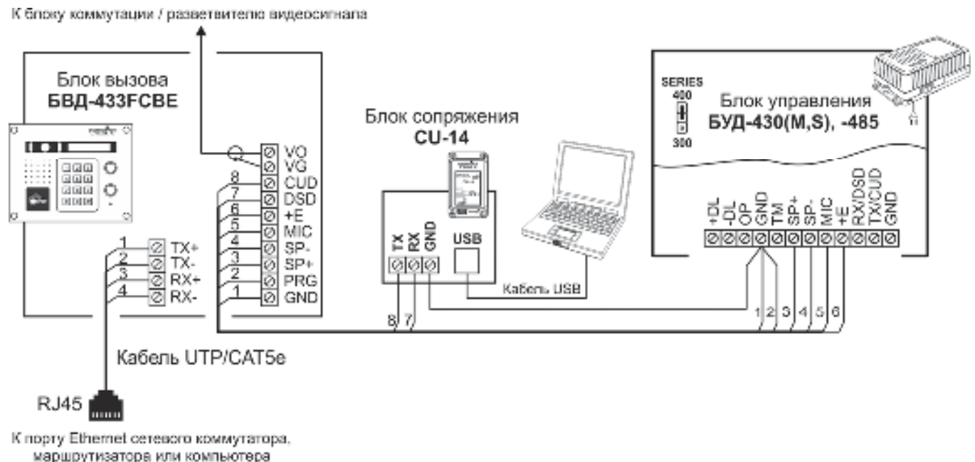
Рисунок 15.1 - Схема соединений блока вызова с блоками управления БУД-430(S, M), -485 и блоком сопряжения CU-14
