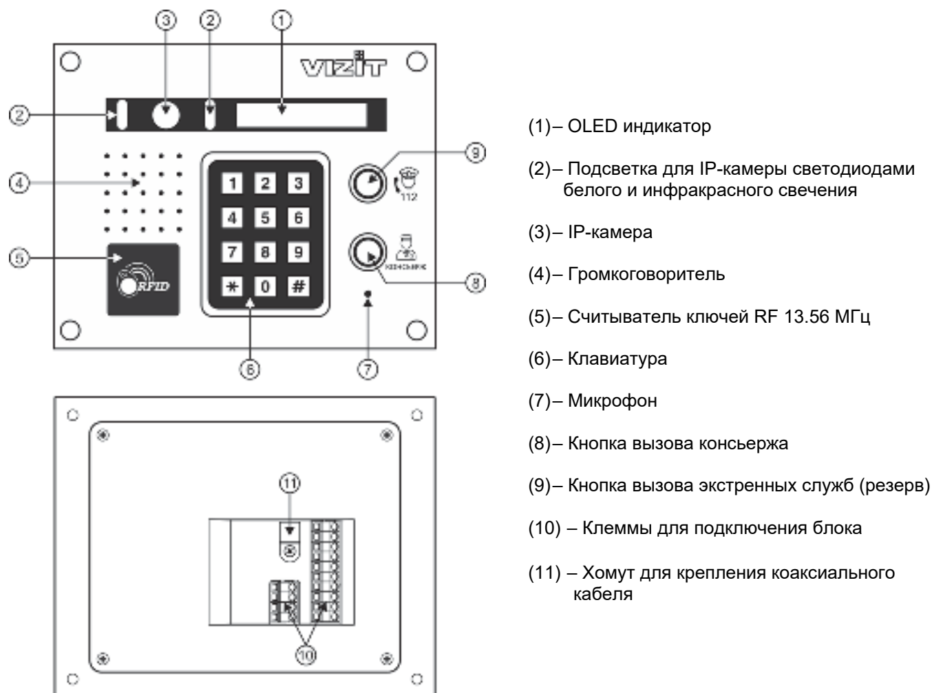
Рисунок 1.1 - Внешний вид блока вызова
