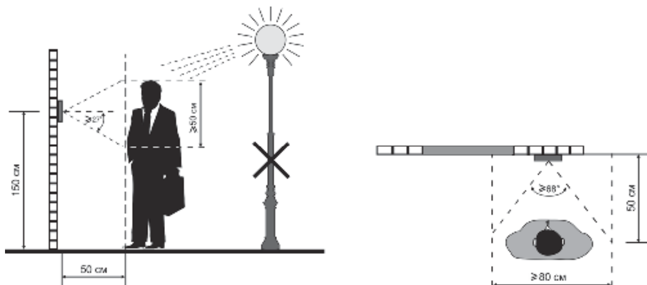
Рисунок 6.1 - Рекомендуемая высота установки блока вызова и область обзора IP-камеры
