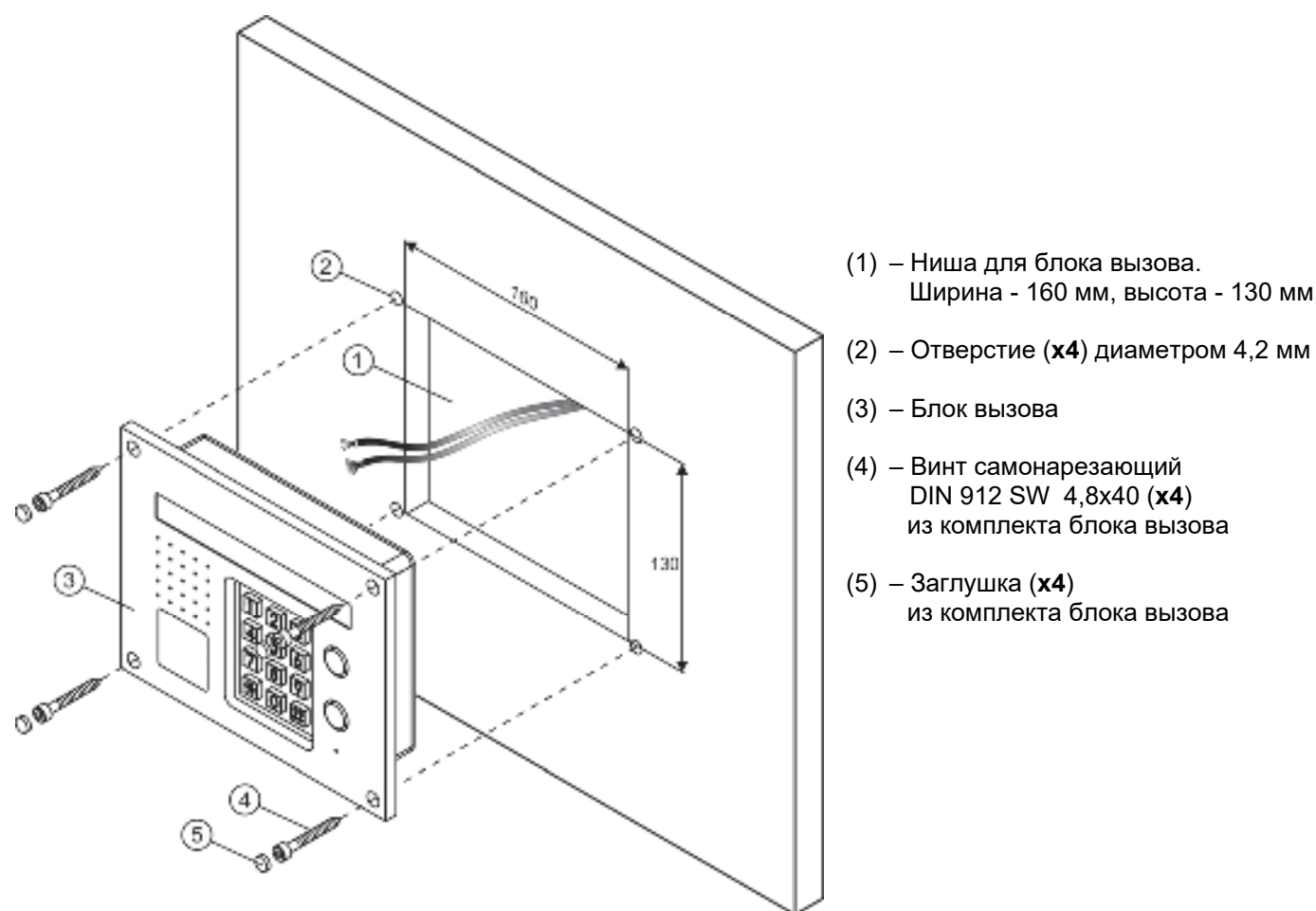
Рисунок 6.2 - Установка блока вызова на неподвижной части металлической двери
