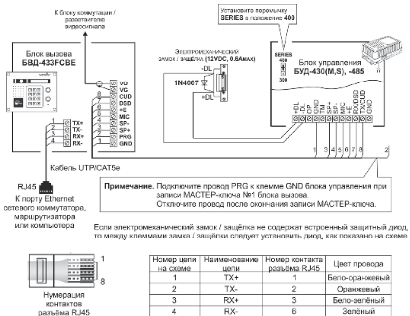
Рисунок 8.3 – Схема соединений блока вызова БВД-433FCBE с блоком управления БУД-430(M,S), -485(M) и электромеханическим замком / защёлкой
