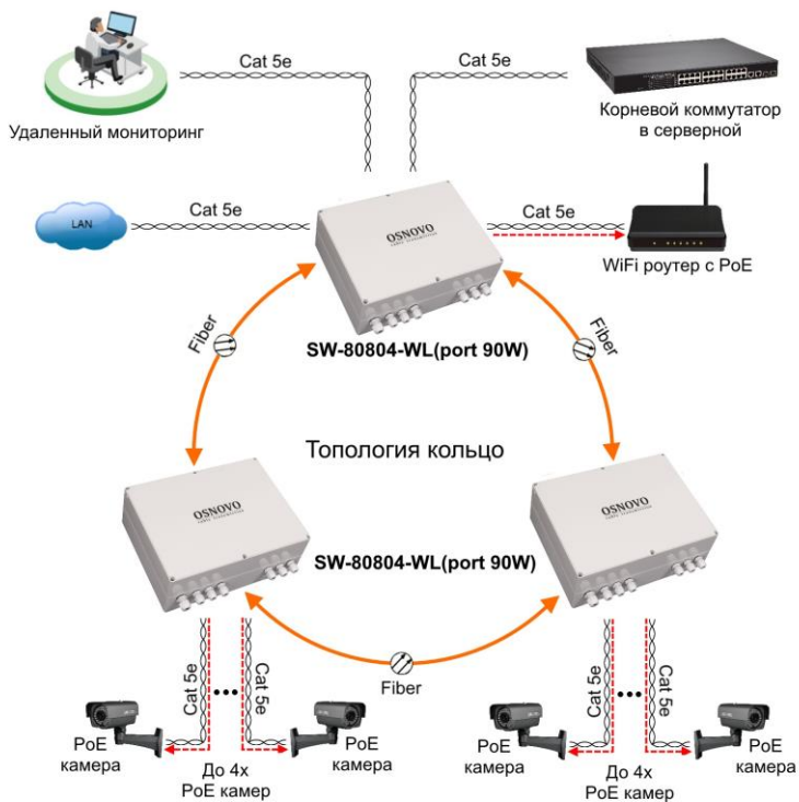
Рис.7 Схема подключения уличного коммутатора SW-80402-WL(port 90W) в топологии «кольцо».
