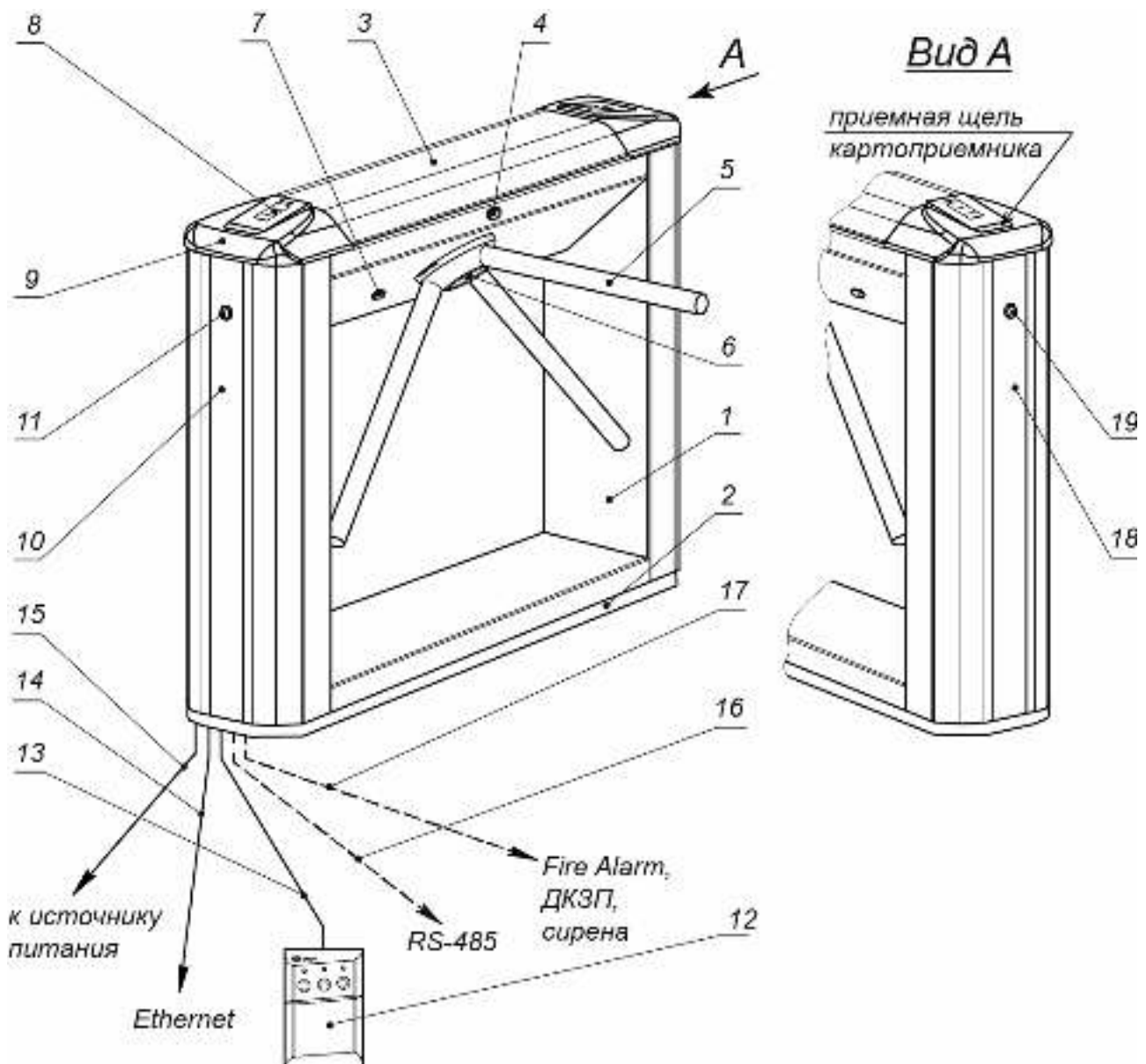
Рисунок 1. Устройство ЭП
