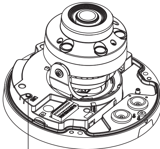
Кнопка «Reset»
