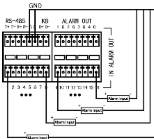
Рис. 2.6. Схема подключения тревожных входов
