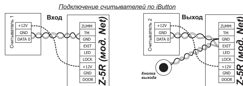
Рис 4. Подключение считывателей.
