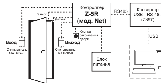
Рис.2 Схема подключения Z-5R (мод. Net).
