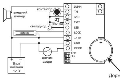
Рис 3. Подключение дополнительных элементов.
