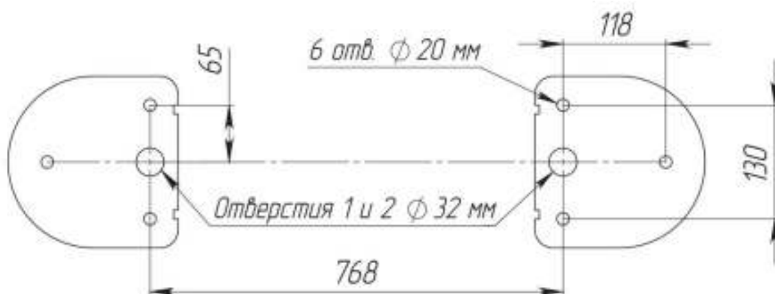
Рис. 5. Установочные размеры
