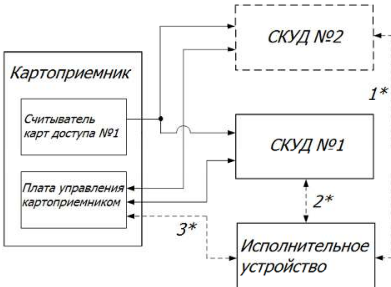
Рис. 19. Структурная схема №2
