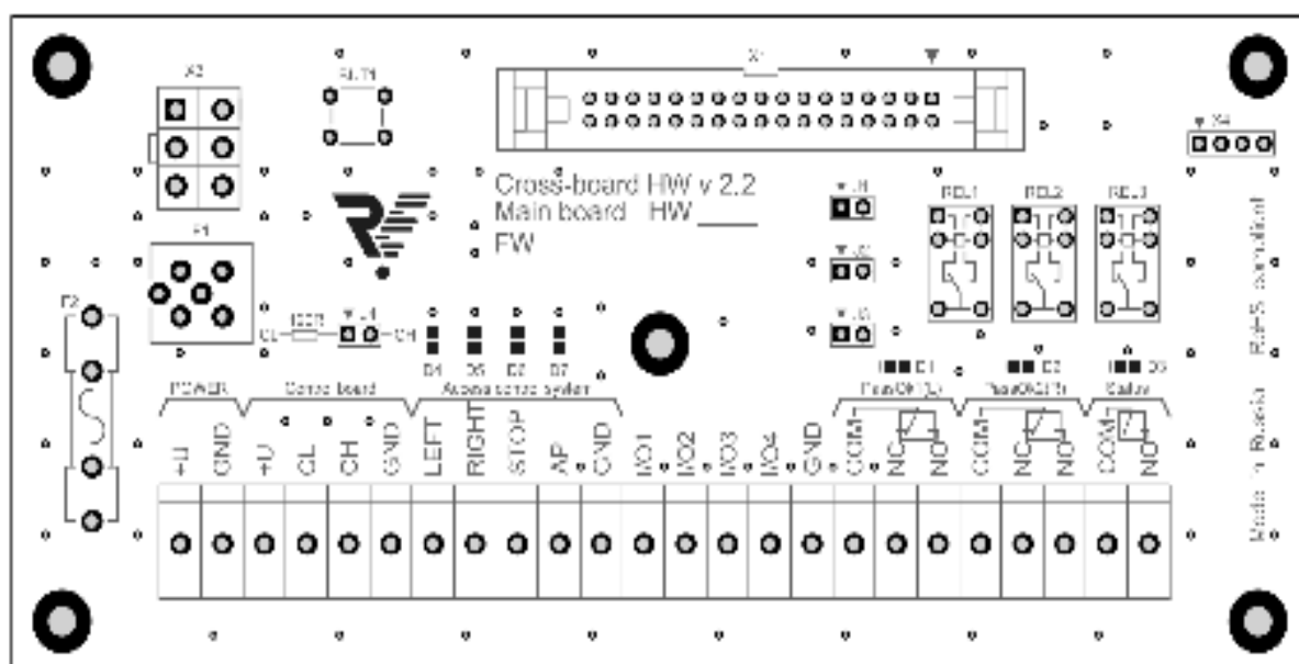
Рис. 8. Внешний вид кросс-платы
