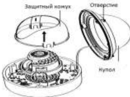
Рисунок 2-1 Снятие купола и защитного кожуха
