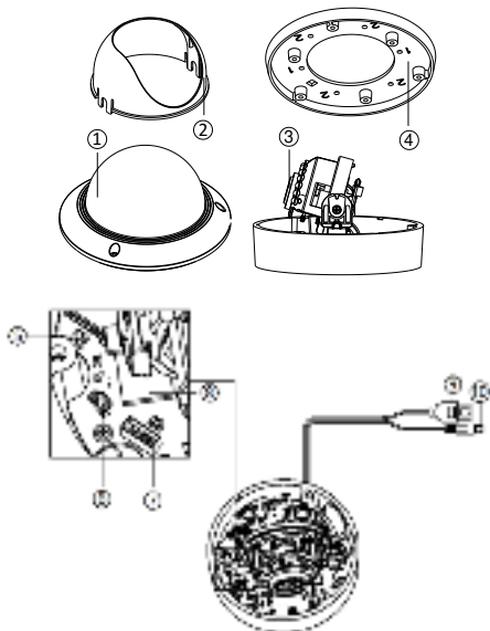
Рисунок 1-1 Купольная камера
