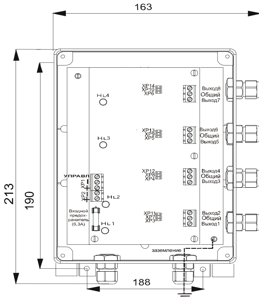
Рисунок 2 -PN-V.8 исп.5
