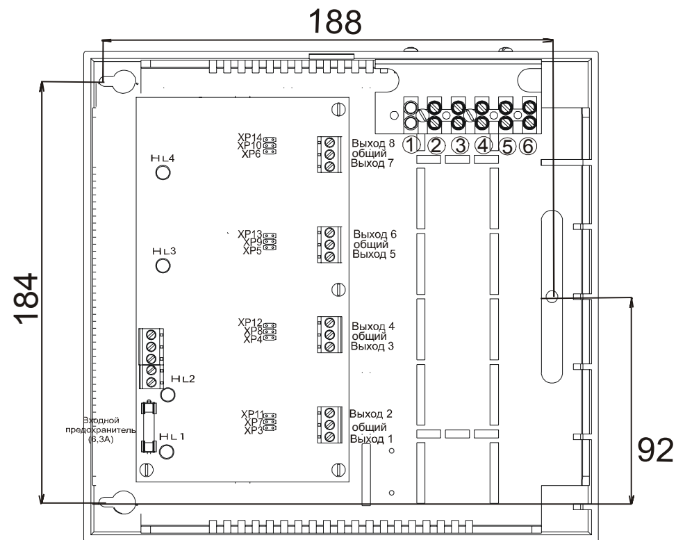
Рисунок 1 - PN-V.8 исп1
