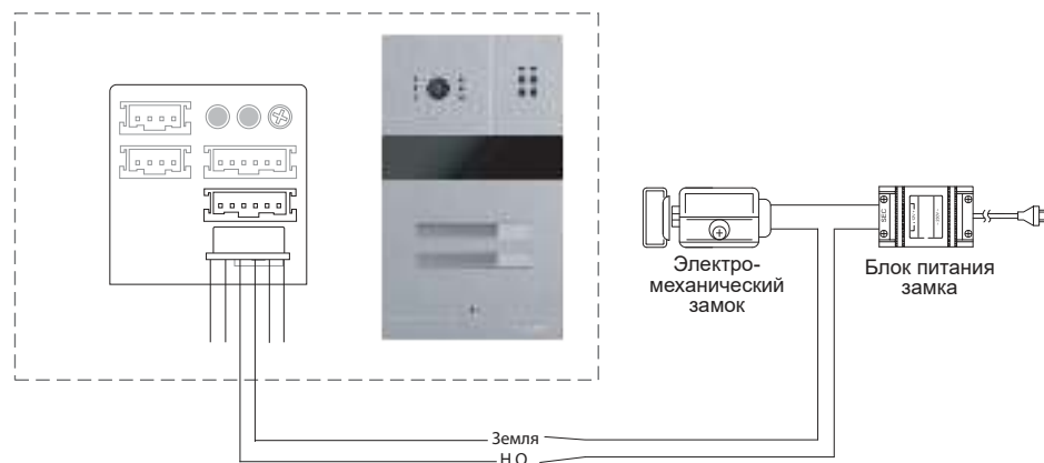
Схема 2. Подключение электромеханического замка к панели МА-02.
