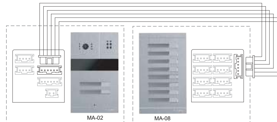
Схема 4. Подключение МА-02 и МА-08.
