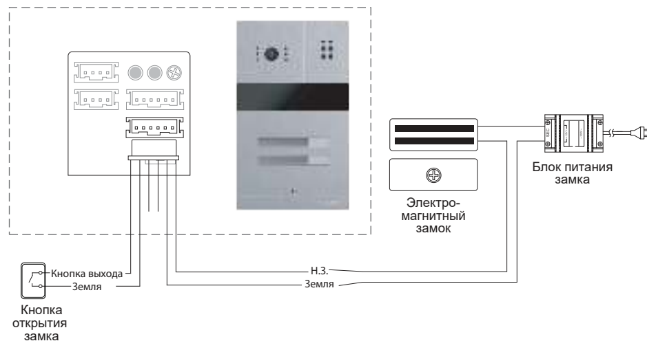
Схема 3. Подключение электромагнитного замка к панели МА-02.
