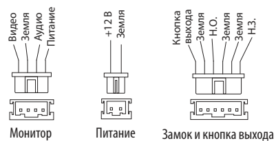
Распиновка разъемов
