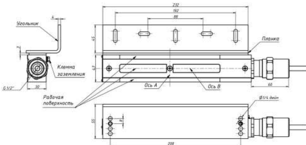
Рис.4 Корпусная часть
