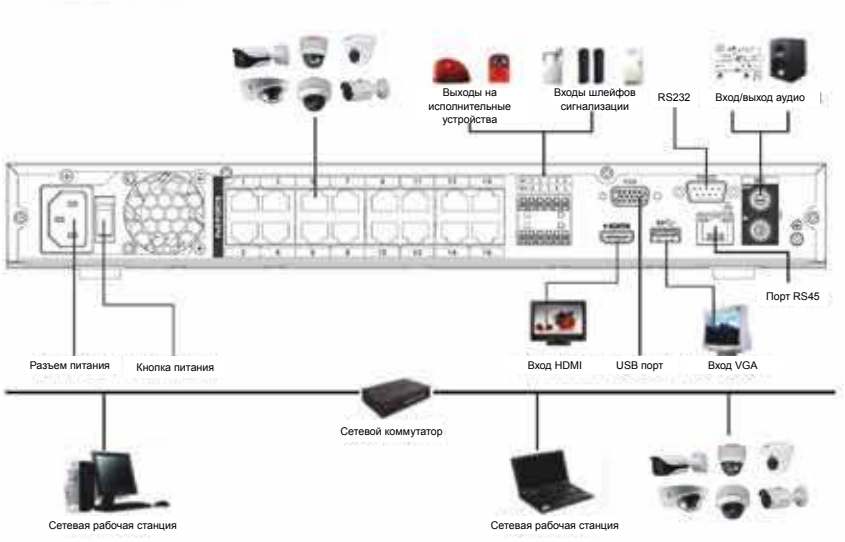
16-канальный NVR
