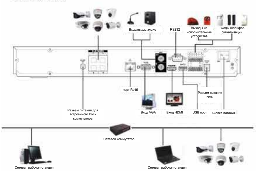
4-канальный NVR
