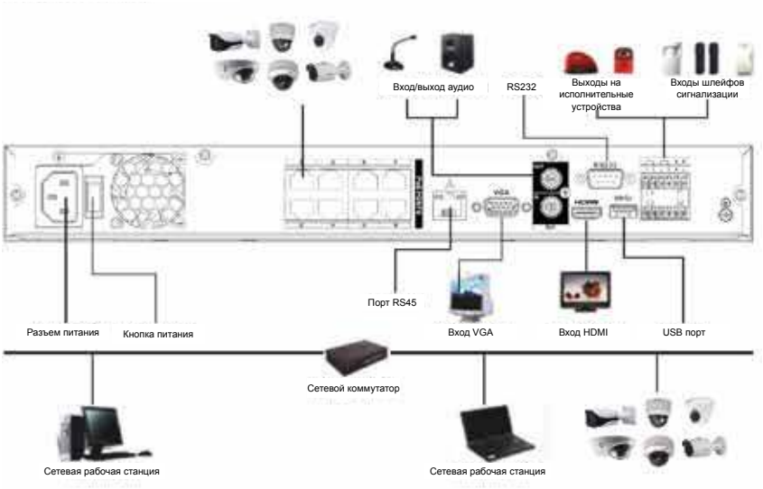
8-канальный NVR
