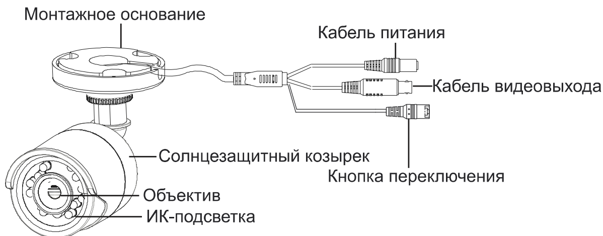
Рис. 1.1. Внешний вид видеокамеры
