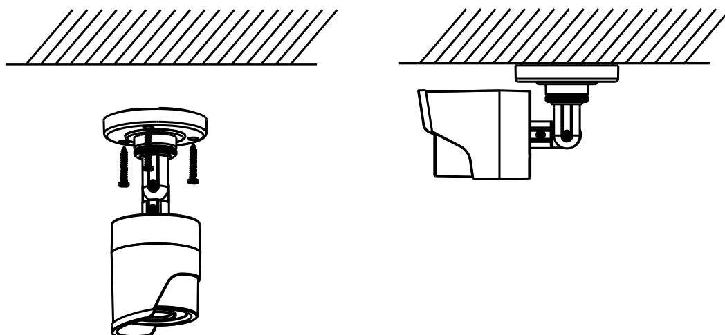
Рис. 2.1. Крепление видеокамеры
