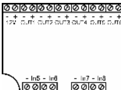
Рисунок 5 – Маркировка клемм верхней платы контроллера
