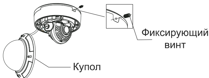
Рис. 5.1. Открытие купола
