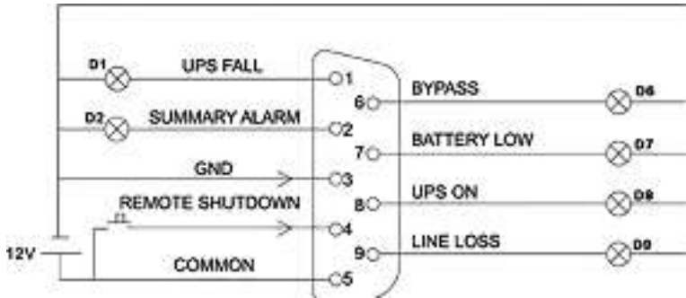
Рис. 11. Отображение состояния ИБП с помощью разъема DB-9
