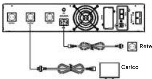
Figura 6. Schema di collegamento per l'UPS da 1000 VA
