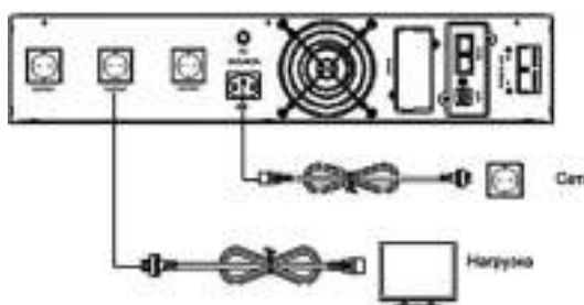
Рис. 6. Схема подключения для ИБП на 1000 ВА
