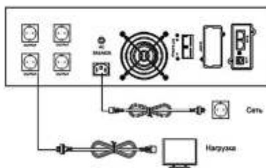
Рис. 7. Схема подключения для ИБП на 1500-3000 ВА
