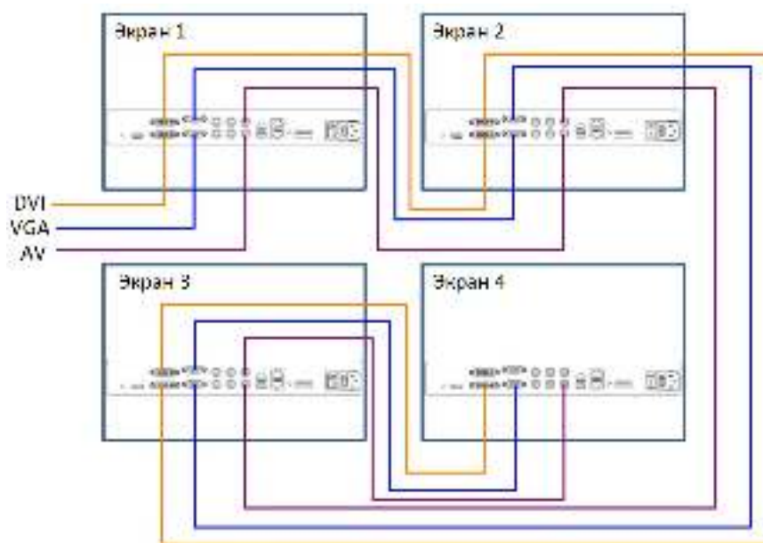
Рисунок 2. 7 Подключение видеосигнала
