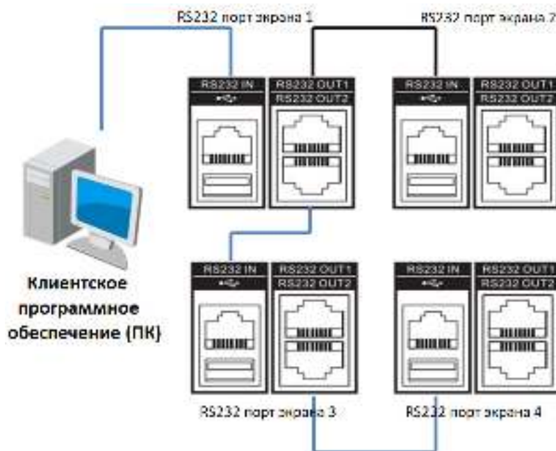
Рисунок 2. 6 Способ подключения
