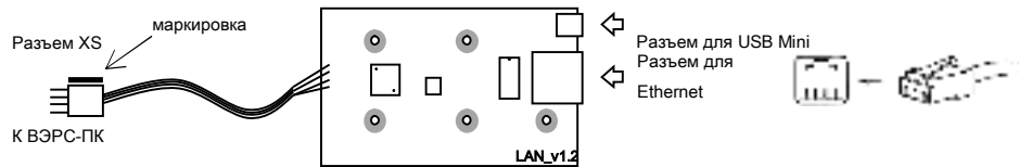
Рисунок 1. Внешний вид Сетевого преобразователя ВЭРС-LAN.
