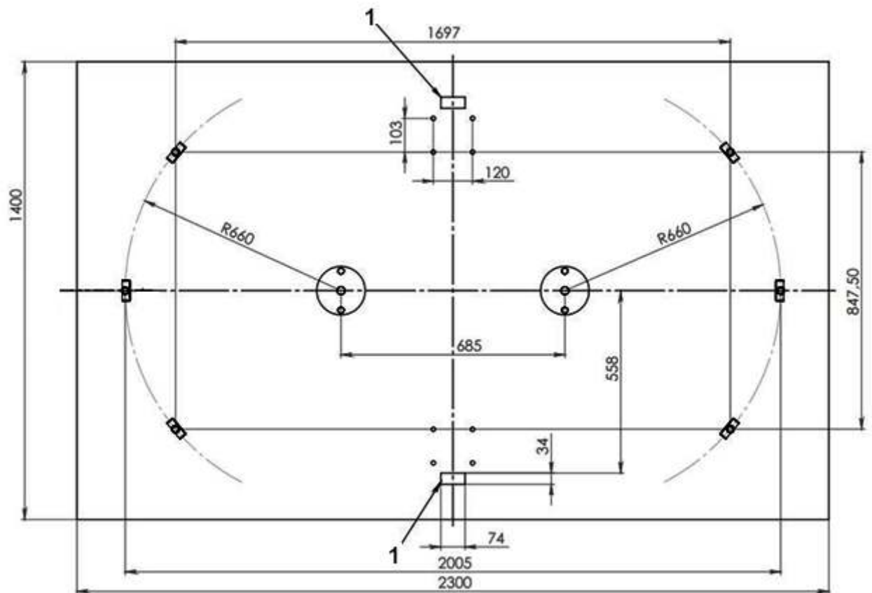
Рисунок 23 – Установочные размеры модификаций турникетов Double pass
