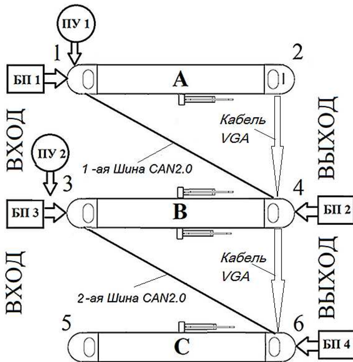
Рисунок 10 – Схема подключения модулей турникета
