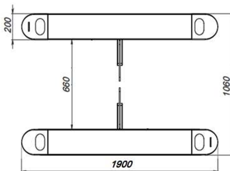
Рисунок 1 – Габаритные размеры турникета
