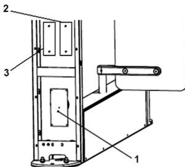
1 - кросс-плата; 2 - плата ИК приемников; 3 - плата ИК передатчиков
