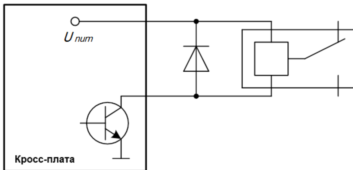
Рисунок 8 – Схема подключения диода параллельно обмотке реле
