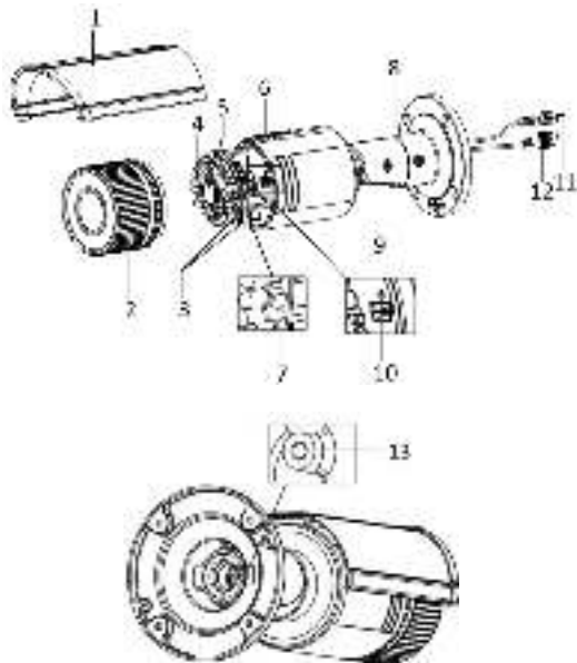
Рисунок 1-1 Цилиндрическая камера
