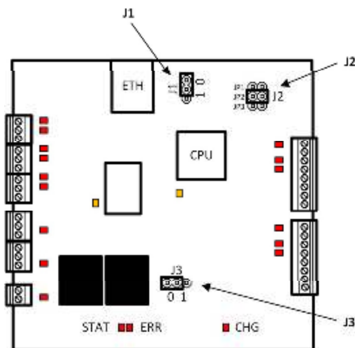
Расположение перемычек на контроллере ST-NC221
