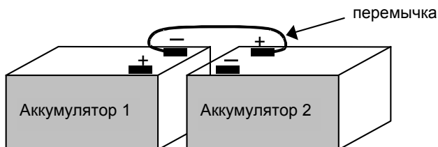
Рисунок 2 – схема последовательного соединения двух аккумуляторов
