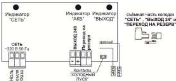
Рисунок 1 - вид изделия с открытой крышкой (схема подключения)
