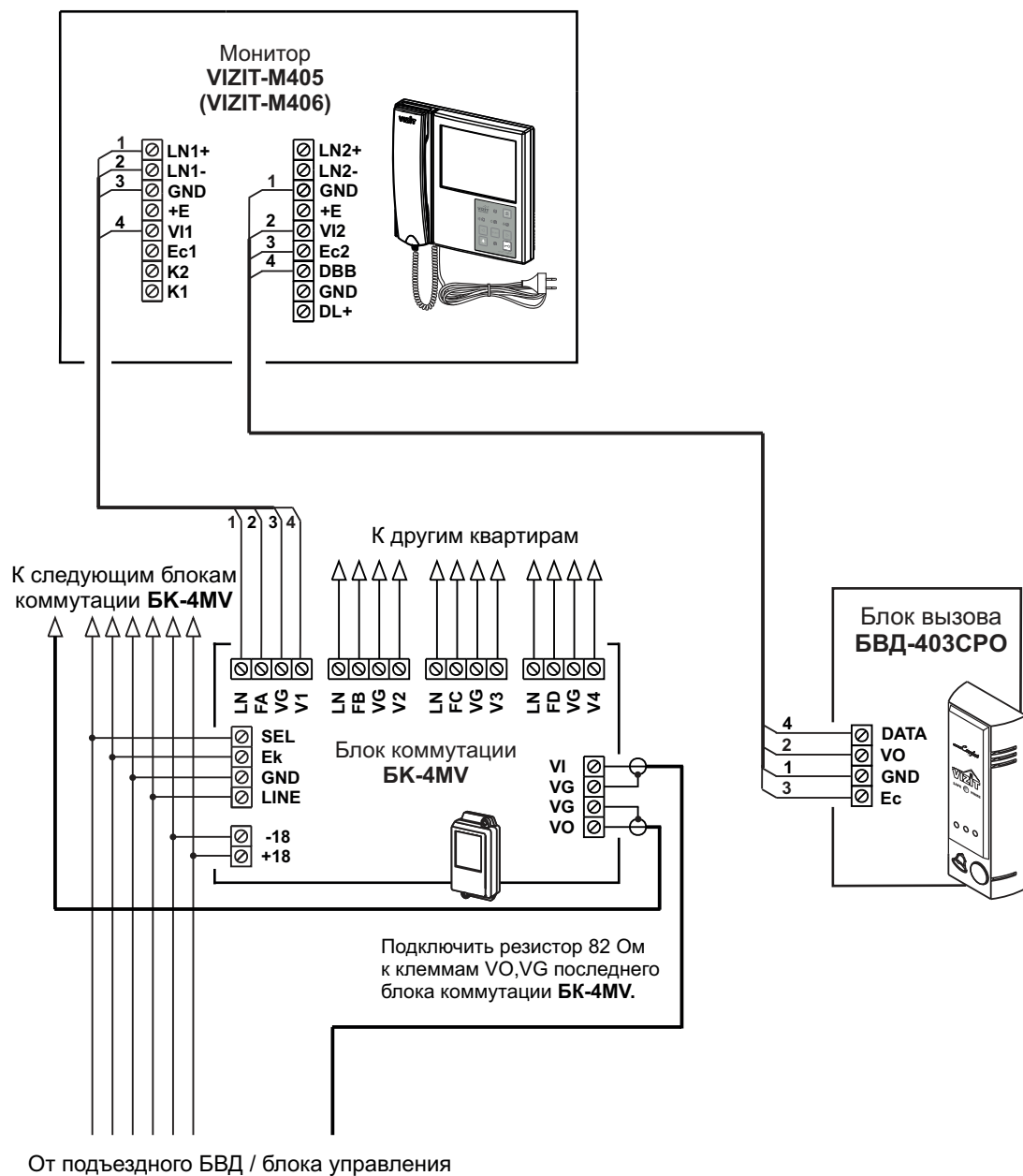
Рисунок 11 - Схема соединений монитора VIZIT-M405 (VIZIT-M406) с блоком коммутации БК-4MV и блоком вызова БВД-403СРО (телекамера + кнопка ЗВОНОК)
