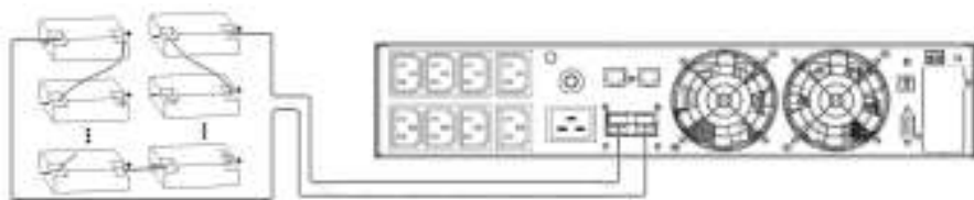
Рисунок 5 – Схема подключения внешних батарей.
