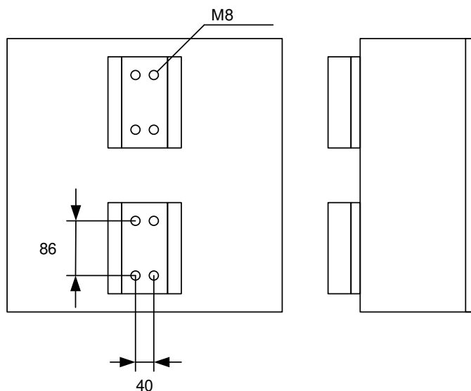
Рис. 5. Установка кронштейна для крепления шкафа на опору
