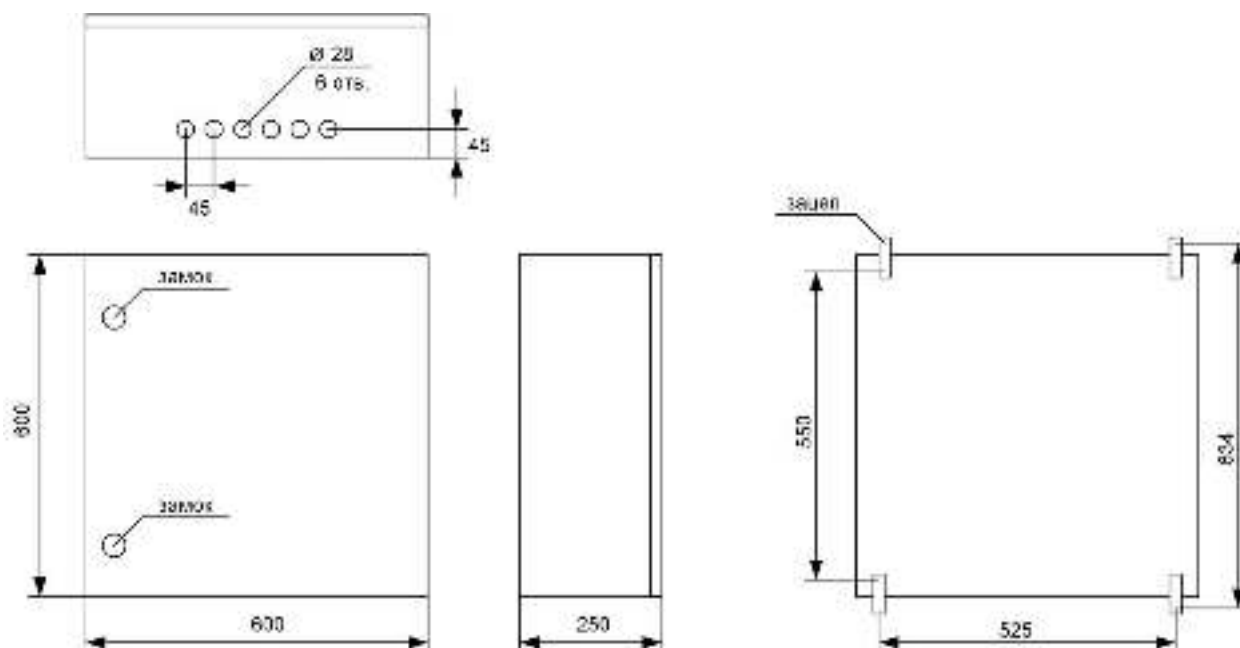
Рис. 8. Чертеж
