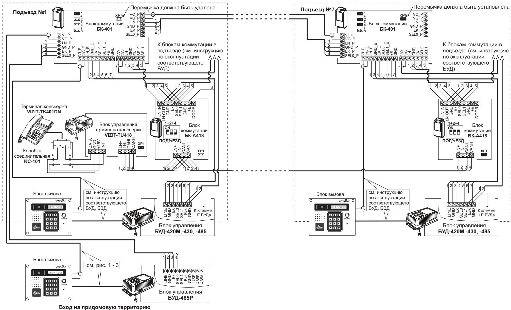
Рисунок 10 - Схема соединений с пультом консьержа VIZIT-PK800
