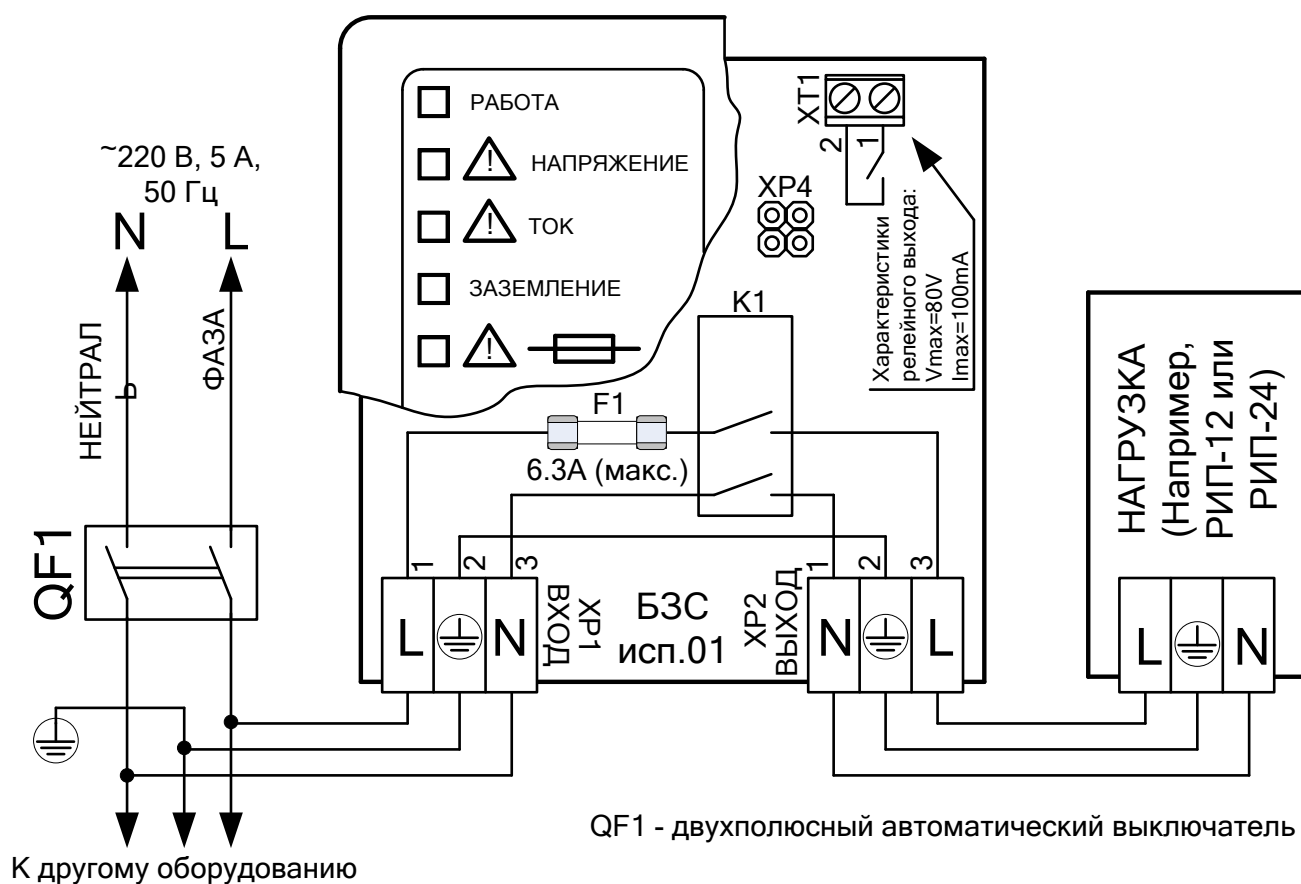
Схема подключения
