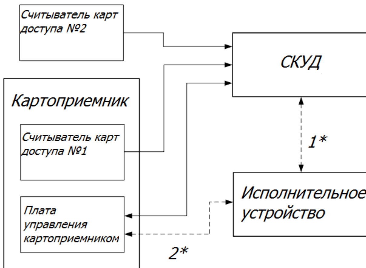
Рис. 20. Структурная схема №1
