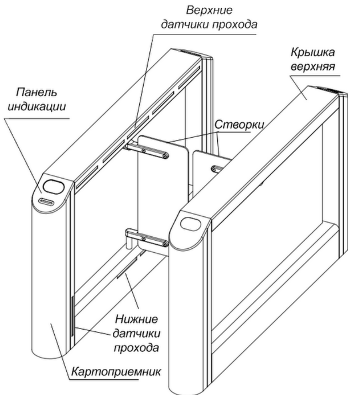
Рис. 1. Общий вид турникета
