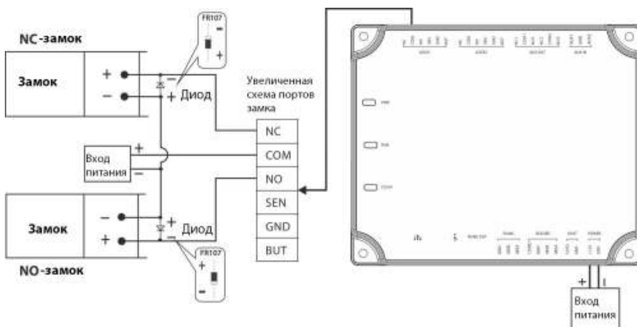
Схема подключения замка
