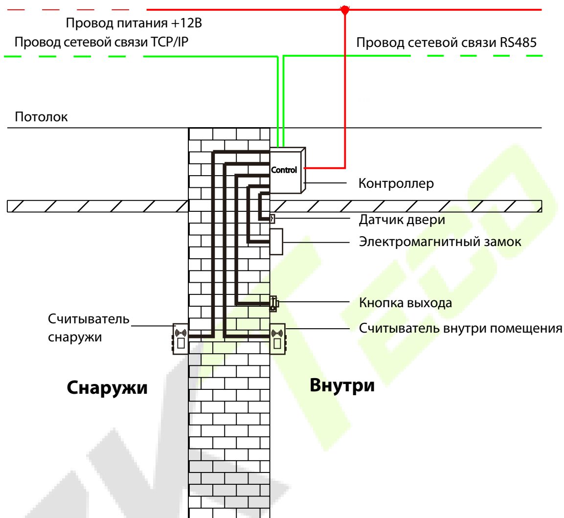
Схема монтажа проводки контроллера доступа
