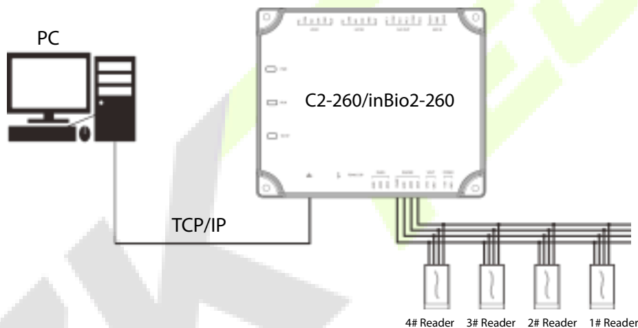
Подключение между контроллером и считывателями карт RS485
