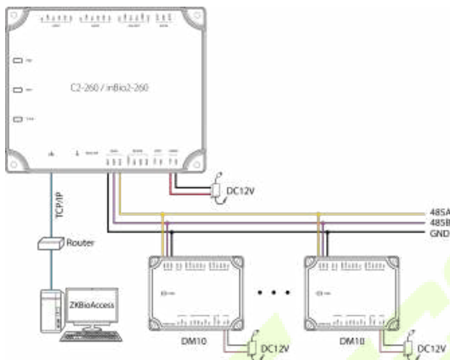
Подключение к DM10 с помощью RS485
