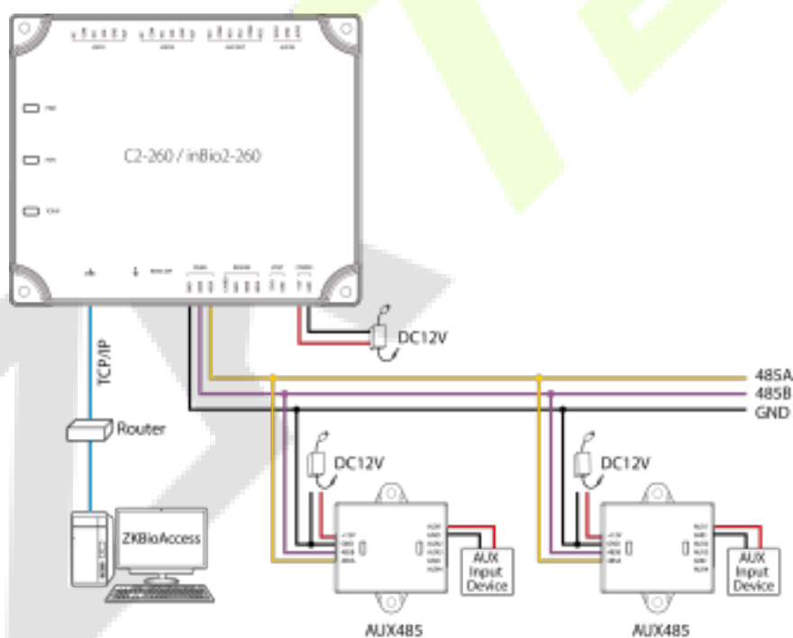
Подключение к AUX485 с помощью RS485
