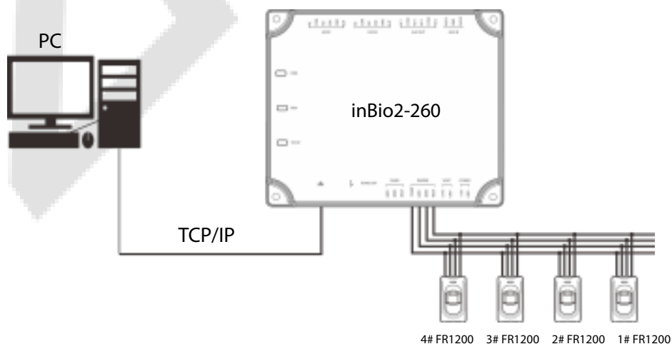
Подключение между контроллером и считывателями отпечатков пальцев
