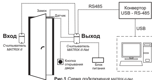
Рис.1 Схема подключения MATRIX-II-Net.
