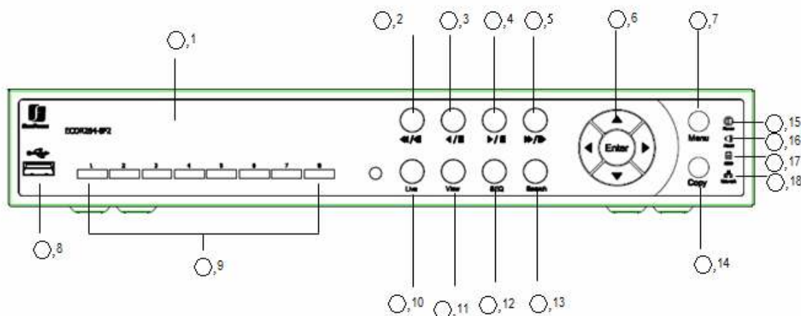
Рисунок 1-1 Передняя панель
