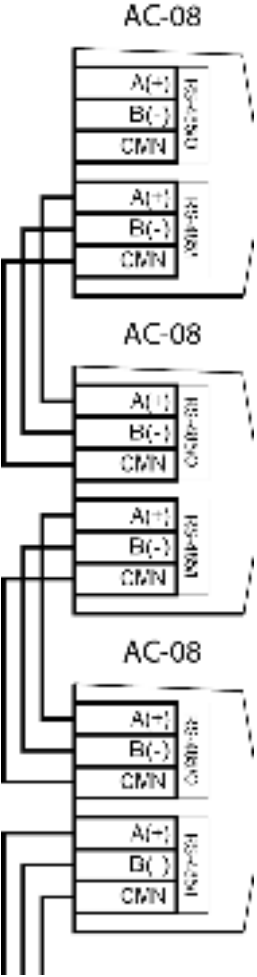
Рисунок 14. Соединение контроллеров по топологии «Шина»
