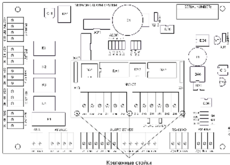
Рисунок 10. Плата контроллера АС-08 с подключенным зонным расширителем NMI-08
