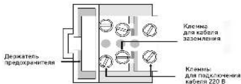
Рисунок 5. Клеммная колодка для кабеля питания
