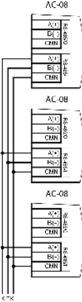
Рисунок 15. Соединение контроллеров по топологии «Звезда»
