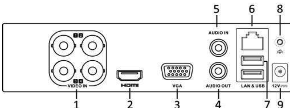
Рис. 1.2. Задняя панель регистратора LTV-RTB-041 00
