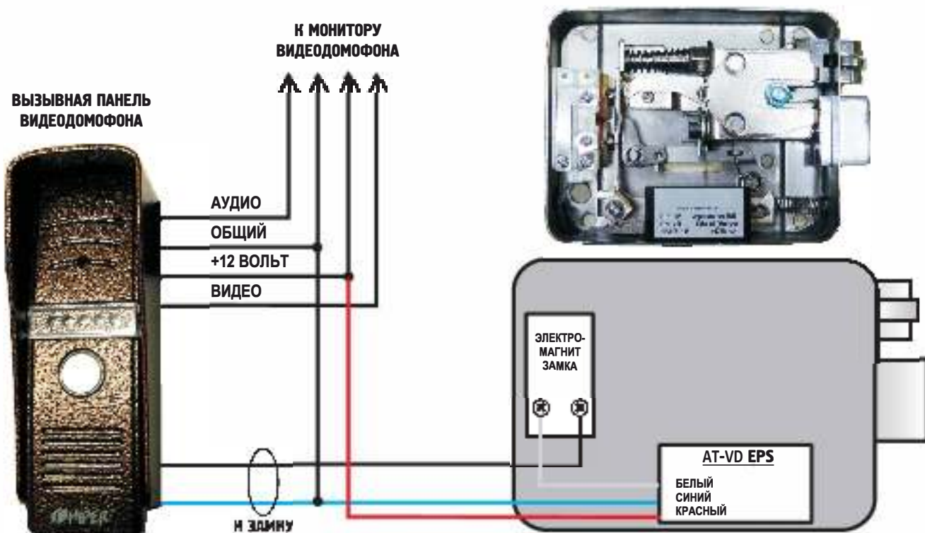
ПРИМЕР С РАЗМЕЩЕНИЕМ УСТРОЙСТВА ВНУТРИ ЗАМКА FALCON EYE
