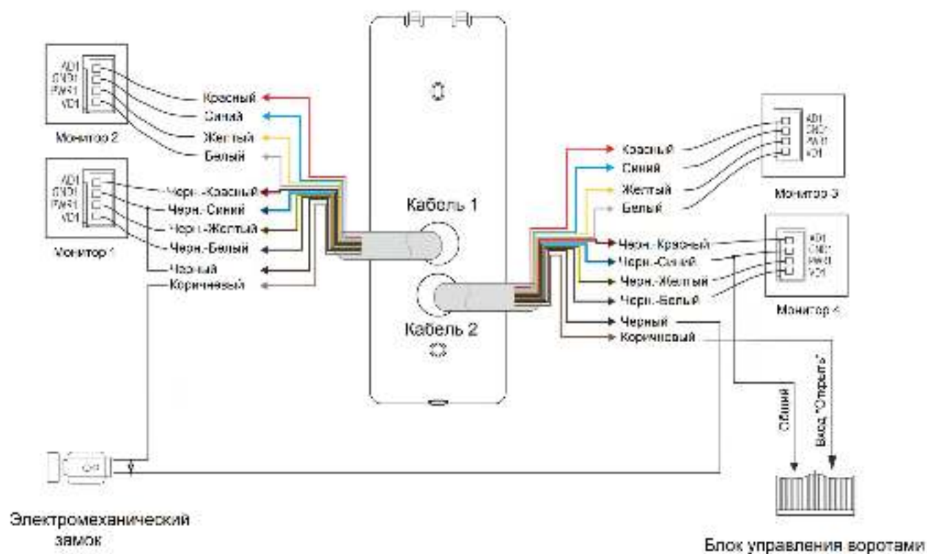
Схема 1 Подключение блока управления воротами и электромеханического замка без использования блока питания:
