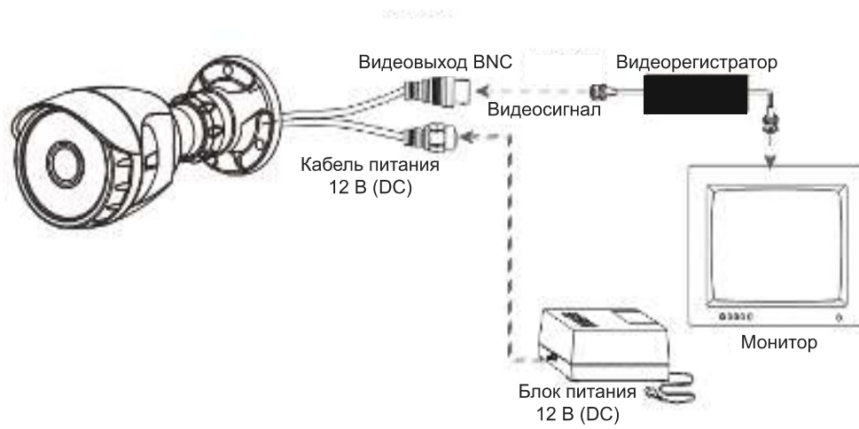
Рис. 2.1. Схема подключения видеокамеры
