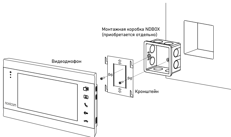
Рис. 5 Монтаж видеодомофона MAGIC 7C
