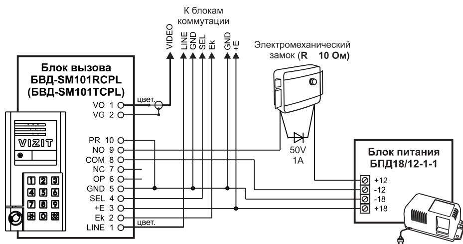
Рисунок 11 - Схема соединений блока вызова БВД-SM101RCPL(TCPL) с электромагнитным замком и блоком питания БПД18/12-1-1
