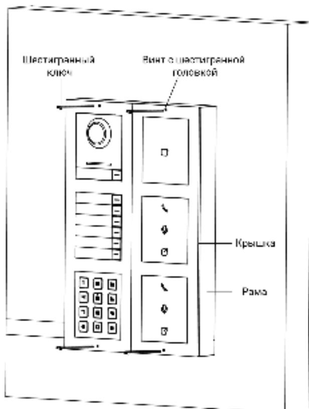
Рисунок 3-52 Фиксация крышки
