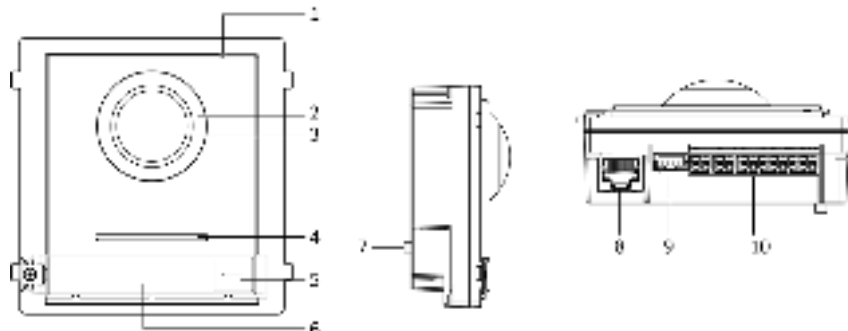
Рисунок 1-1 Внешний вид вызывной панели CTV-IP-UCAM
