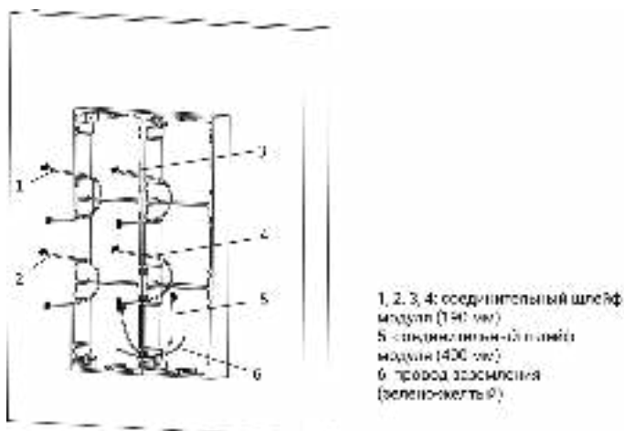
Рисунок 3-48 Размещение коммутационных кабелей и шлейфов
