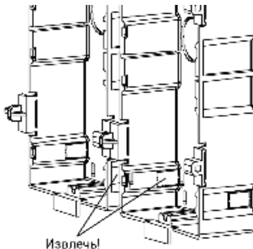
Рисунок 3-56 Удаление пластиковых вставок
