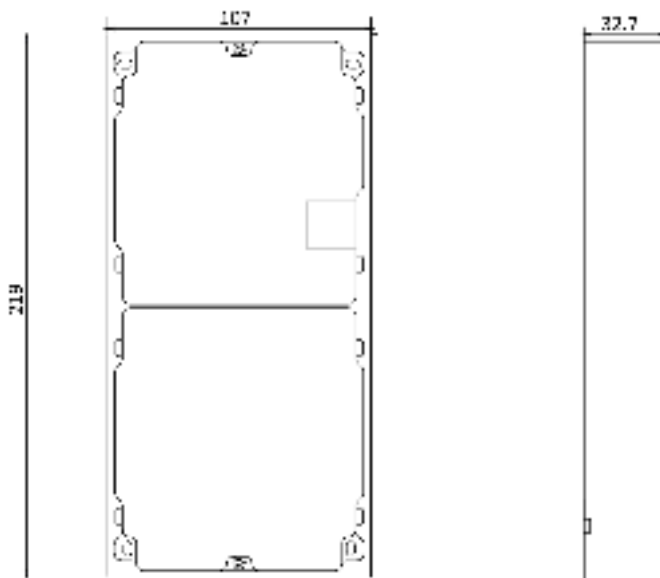
Рисунок 3-15 Монтажная рамка
