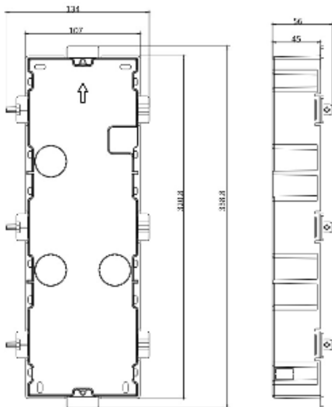
Рисунок 3-53 Монтажная коробка
