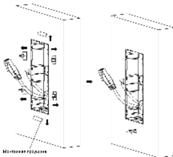
Рисунок 3-26 Извлечение монтажных проушин
