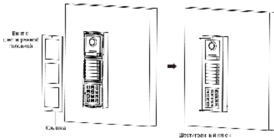
Рисунок 3-36 Фиксация крышки
