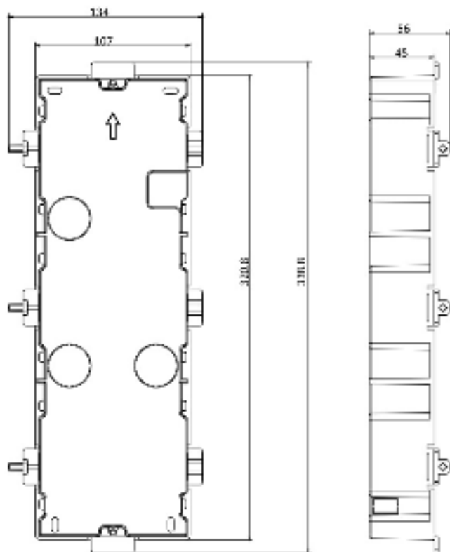
Рисунок 3-37 Монтажная коробка
