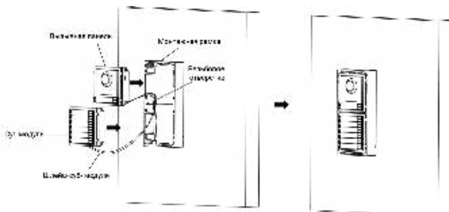
Рисунок 3-20 Установка вызывной панели и субмодуля
