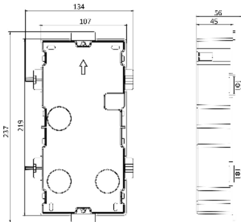
Рисунок 3-22 Монтажная коробка
