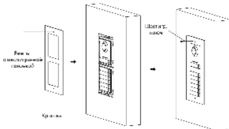
Рисунок 3-28 Фиксация крышки
