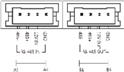
Рисунок 2-2 Разъем дополнительного модуля
