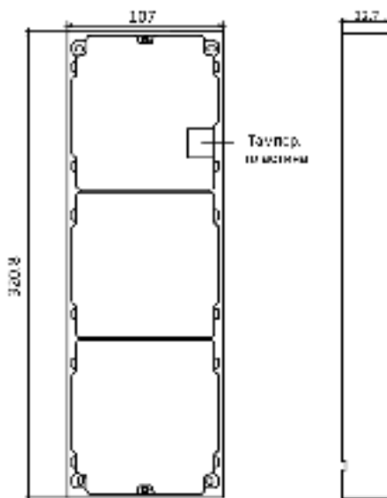
Рисунок 3-44 Монтажная рамка
