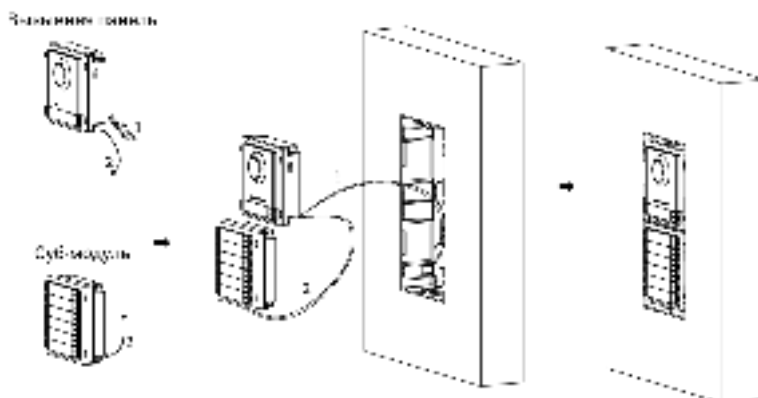
Рисунок 3-27 Подсоединение кабелей и установка модулей
