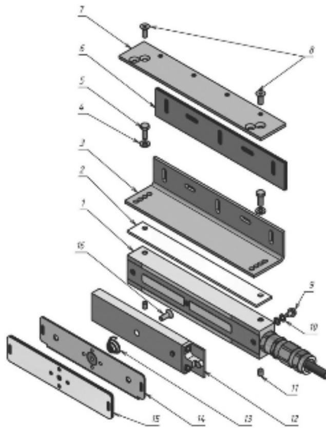
Рисунок 1- Комплект поставки
