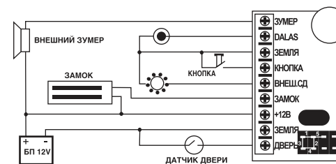
Рис.2 Схема подключения.
