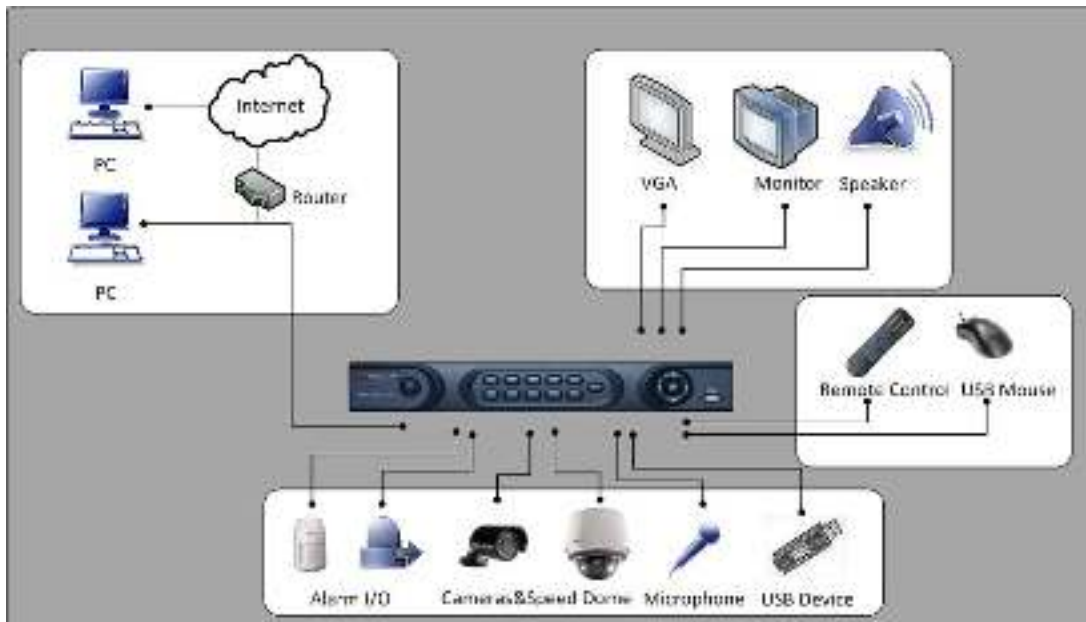
Рис.6. Подключение устройства
