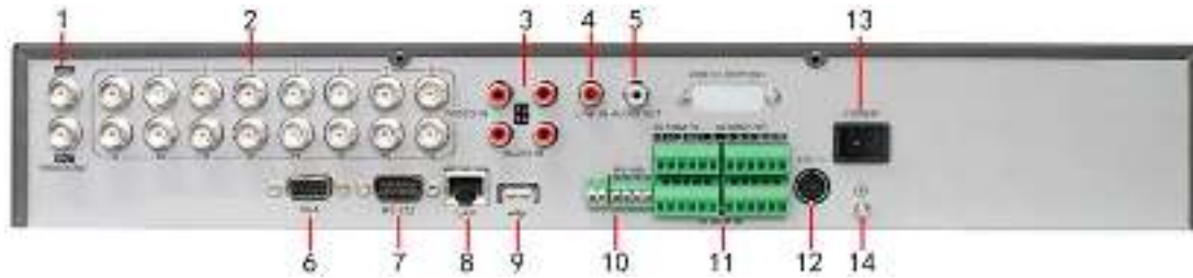
Figure 17. Задняя панель DS-7216HVI-ST
