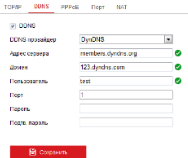
Рисунок 7-2 Настройка DynDNS
