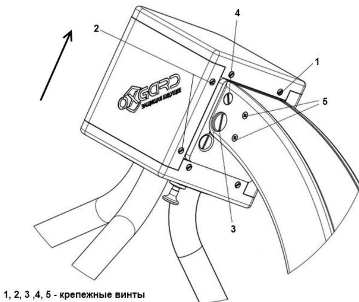
Рисунок 10 – Демонтаж защитного кожуха
