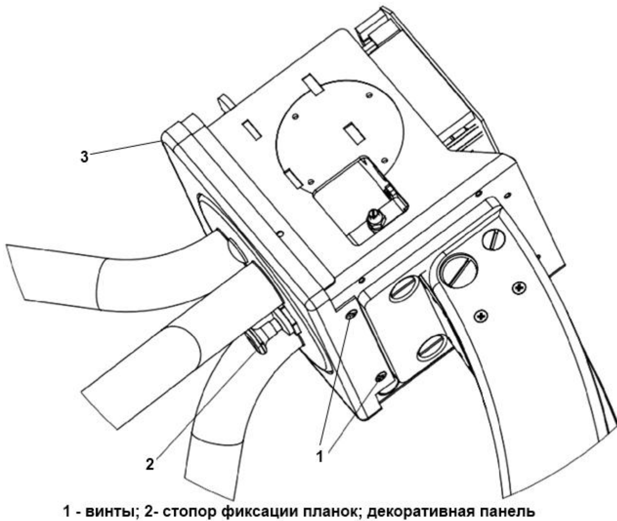
Рисунок 11 – Демонтаж декоративной панели
